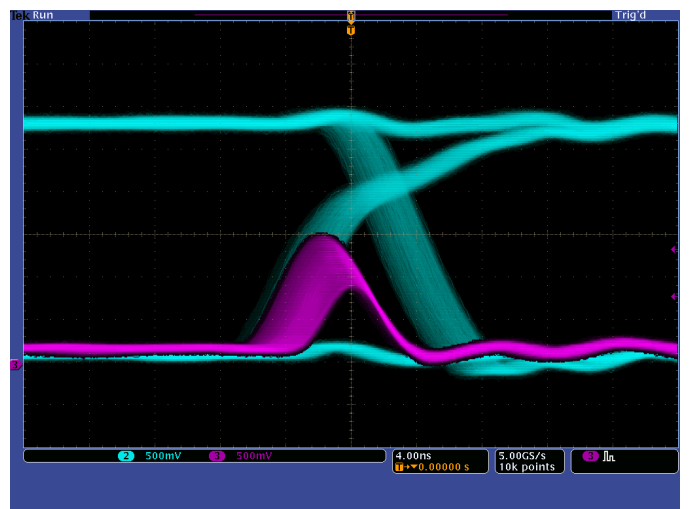
디지털 포스퍼 기술은 50,000wfms/s 을 넘는 파형 캡처 속도와 실시간 밝기 그레이딩을 가능하게 합니다.
