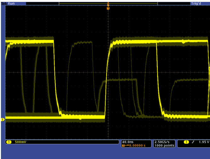
발견 - 50,000wfms 가 넘는 빠른 파형 캡처 속도 덕분에 식별하기 어려운 글리치 및 기타 간헐적인 이벤트를 캡처할 가능성이 높아집니다.
