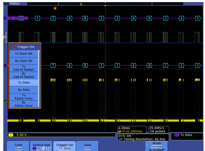
캡처 - RS-232 버스를 지나는 특정 전송 데이터 패킷에서의 트리거입니다. 특정 시리얼 패킷 내용 트리거 등의 완전한 트리거 세트를 통해 관심 있는 이벤트를 빠르게 캡처할 수 있습니다.
