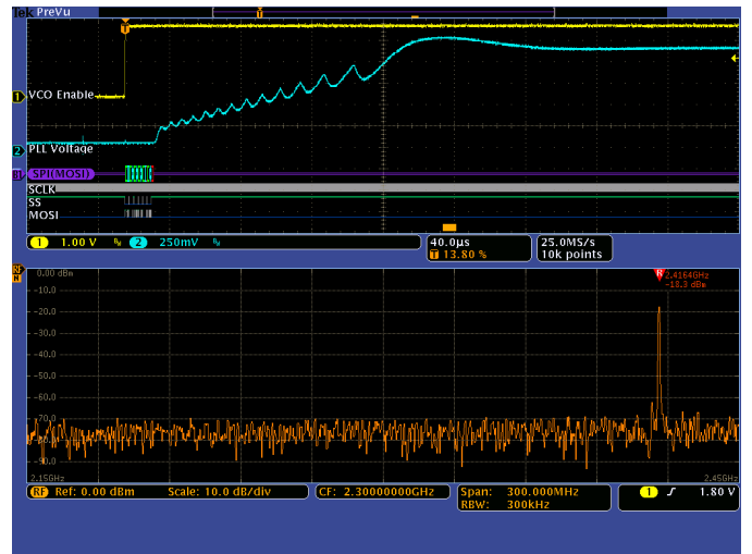
그림 3 - 스펙트럼 시간(Spectrum Time)이 오른쪽으로 다시 120µs 만큼 이동했습니다. 이때 스펙트럼은 PLL 이 실제로는 올바른 주파수를 넘어서서 2.4164GHz 까지 이동했음을 보여줍니다.
