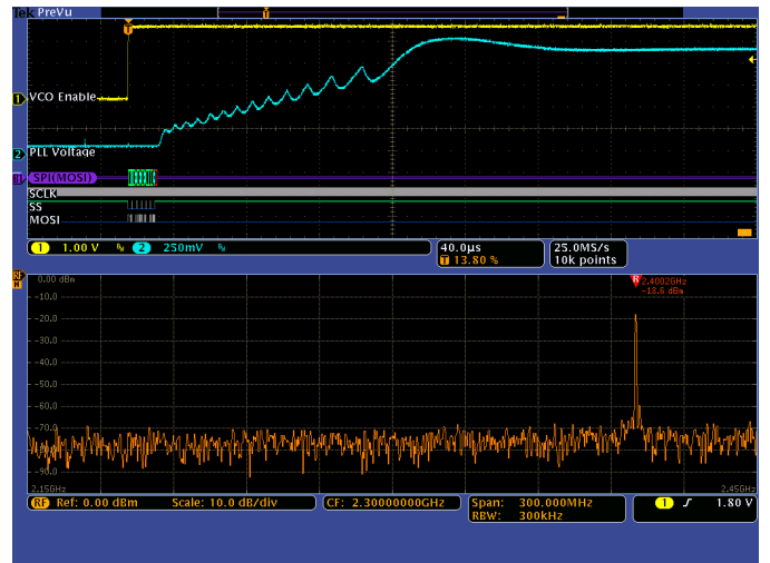
그림 4 - PLL 이 결국 올바른 주파수인 2.400GHz 에 도달했습니다. VCO 가 활성화된 지 340µs 후입니다.
