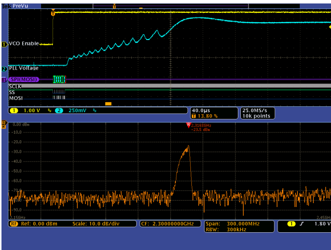
그림 2 - 스펙트럼 시간(Spectrum Time)이 오른쪽으로 약 60µs 이동했습니다. 이때 스펙트럼은 PLL 을 올바른 주파수(2.400GHz)로 조정 중임을 나타냅니다. 2.3168GHz 까지 조정된 상태입니다.
