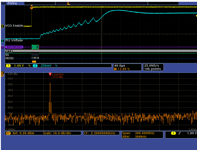
그림 1 - PLL 커짐을 표시하는 시간 및 주파수 도메인 보기입니다. 채널 1(노란색)은 VCO 를 활성화하는 컨트롤 신호를 프로빙합니다. 채널 2(하늘색)는 VCO 조정 전압을 프로빙합니다. 원하는 주파수로 PLL 을 프로그래밍하는 SPI 버스는 디지털 채널 세 개로 프로빙되고 자동적으로 디코딩됩니다. 스펙트럼 시간이 VCO 가 활성화된 후 배치되었고 PLL 에 적정 주파수인 2.400GHz 를 알려 주며 SPI 버스의 명령과 일치 하고 있습니다. 회로가 켜져 있을 때 RF 는 2.2202GHz 상태입니다.
